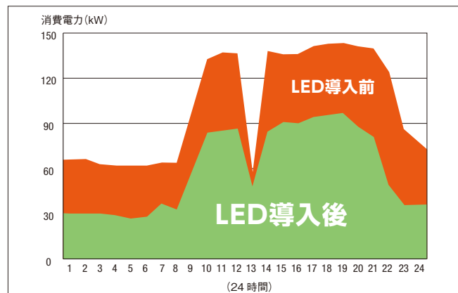
LED導入による電力消費量の比較
