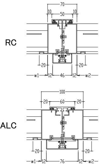
分解方立
