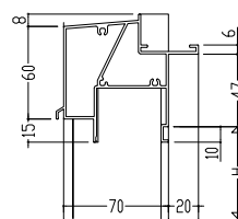
アスロック対応上枠
